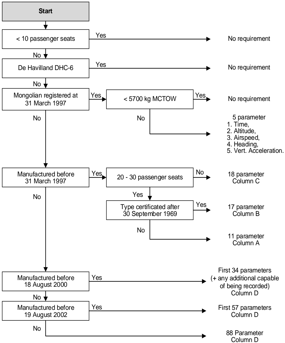
Зураг 1. FDR тодорхойлох бүдүүвч
